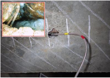
ファイバースコープによる空洞調査
