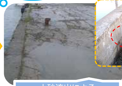
土砂流出によるエプロンの沈下・陥没
